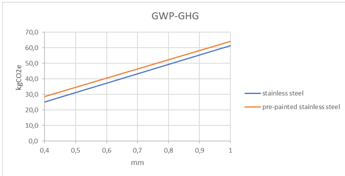
GWP-GHG variazioni con diversi spessori e finiture dell'acciaio
